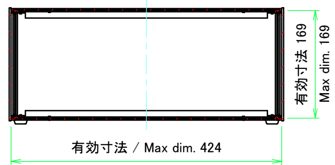
C-C ( 1 : 6 )
