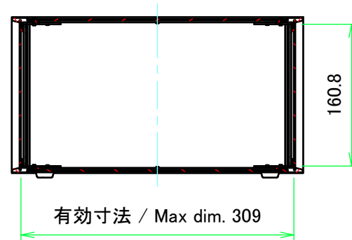
A-A ( 1 : 6 )
